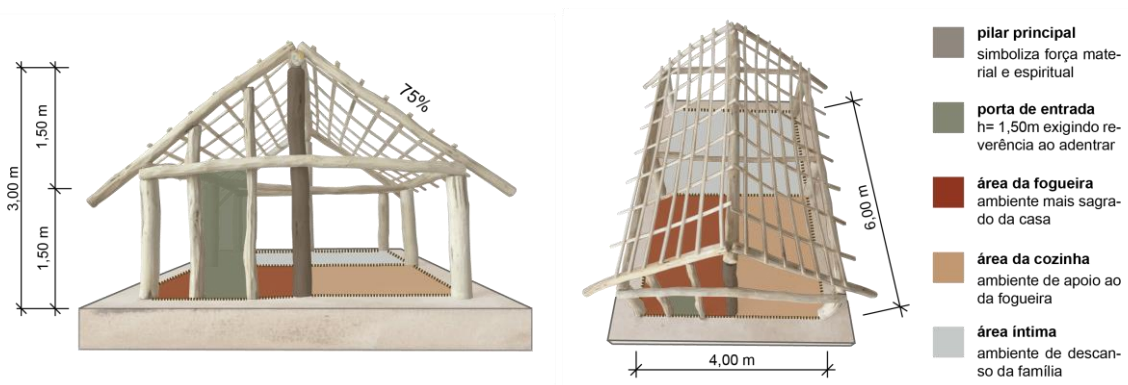
Figuras 6 e 7: Maquete Oga Tradicional.
