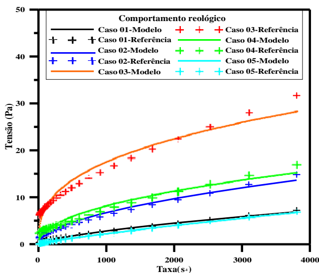
Gráfico 01: Resultados do estudo de reologia das polpas para validação do método: relação entre taxa e tensão de cisalhamento
